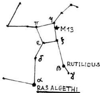
Sohvězdí Herkula
